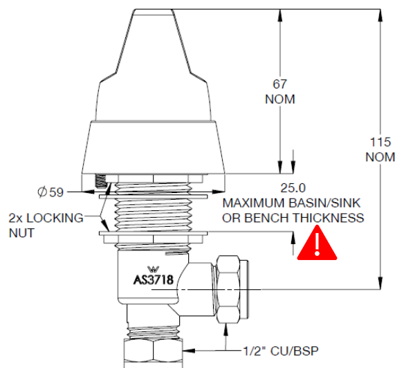
Ezy-Grip Assembly
